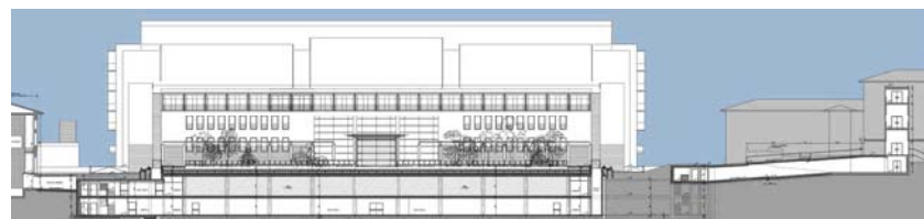
SEZIONE TRASVERSALE
