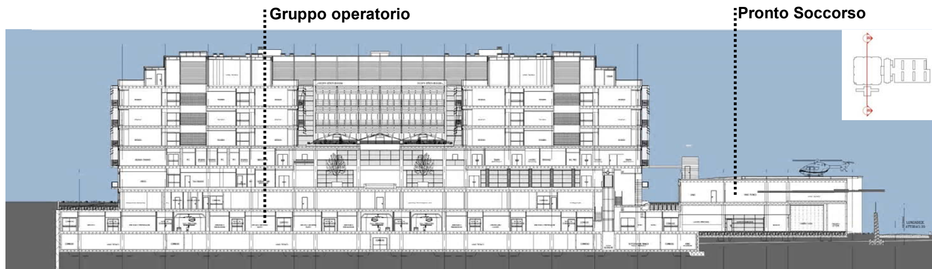
SEZIONE TRASVERSALE
